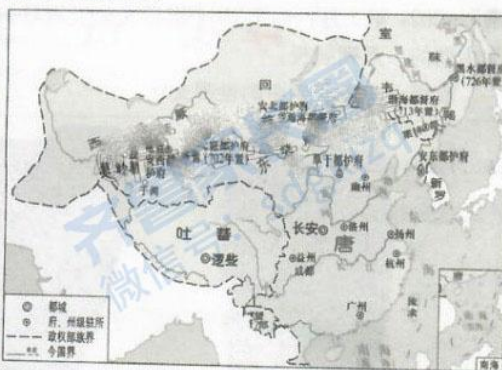
▲ 唐朝前期疆域和边疆各族的分布图 (669年)
