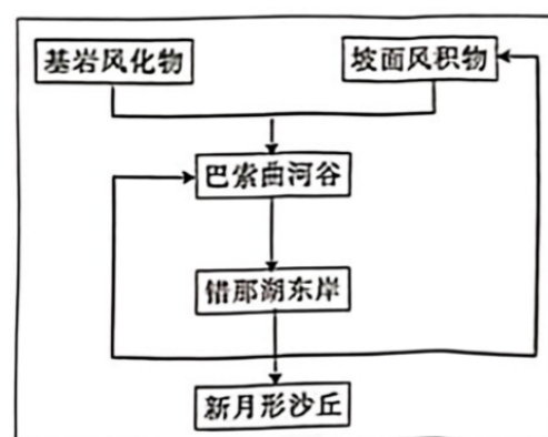
沙丘形成机制示意图
