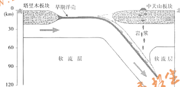
图6为我国新疆南部的板块运动示意图。读图, 回答第11题。
