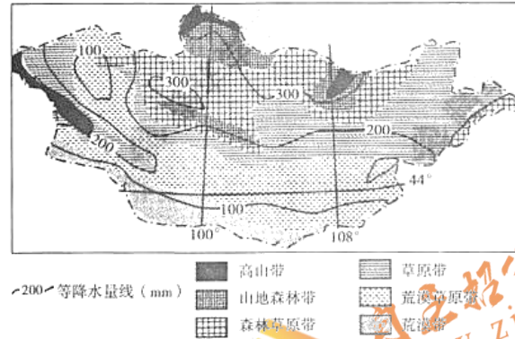
图5为某国等降水量线和自然带分布图。读图,回答第9、10题。
