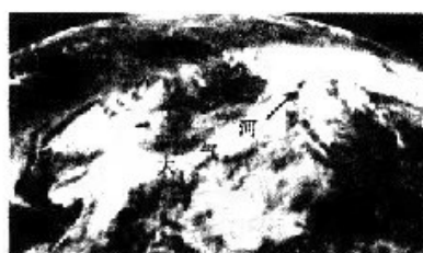
图甲 “大气河”位置图
