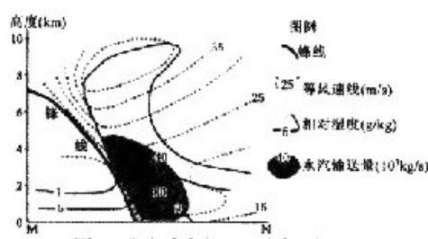
图乙 北半球大气河垂直剖面示意图
