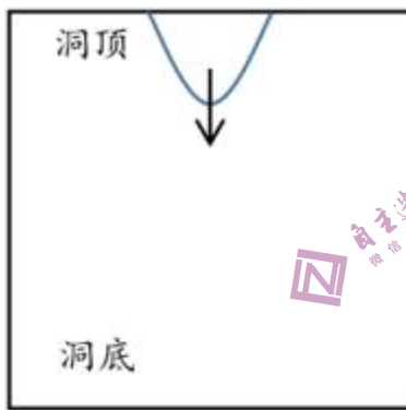
石钟乳
