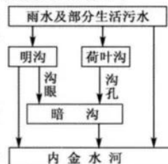
紫禁城地下排水示意图
