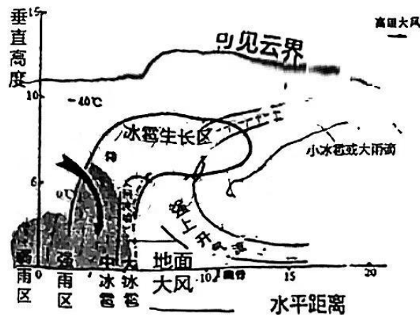
积雨云结构示意图（单位：公里）
