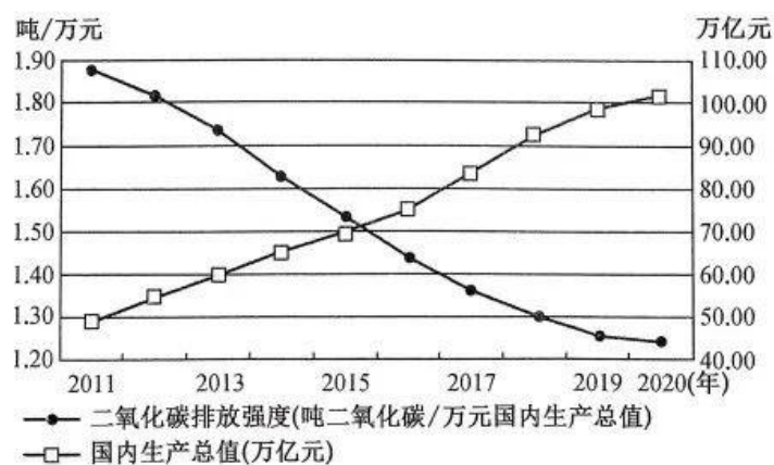
2011~2020 年我国二氧化碳排放强度和国内生产总值的变化情况
