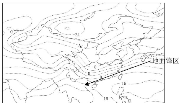
P_3 等压面
