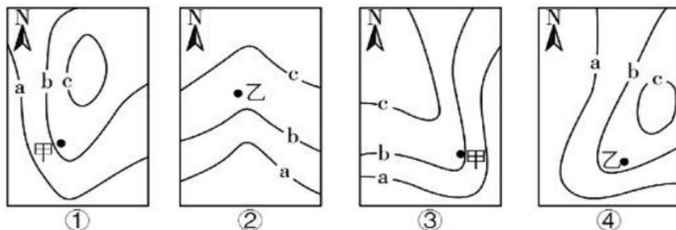
图例 a 等压线 数值 a>b>c
