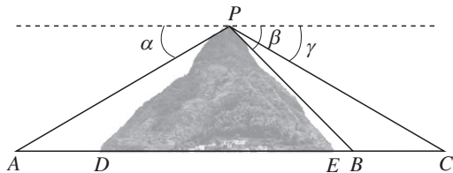
图 33 计算隧道长度示意图
