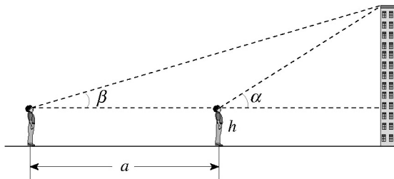
图 12 两次测角法示意图
